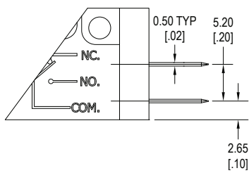
SPST N.O.
